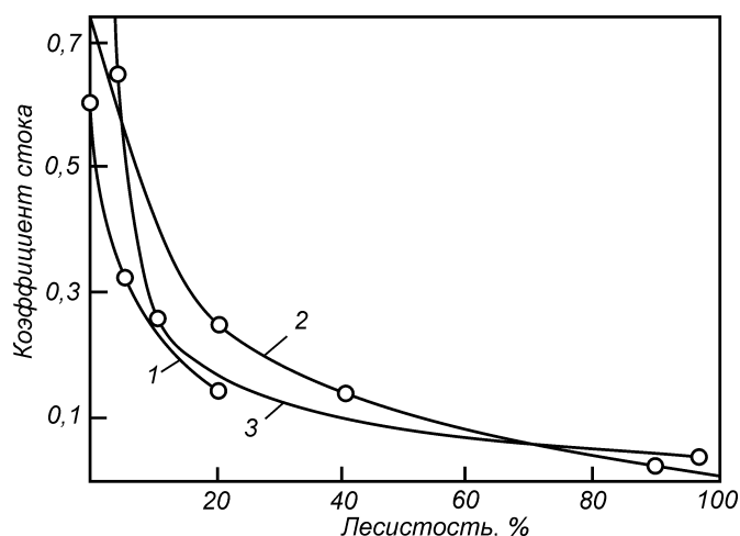
Рис. 12. Изменение поверхностного стока в зависимости от лесистости территории:
