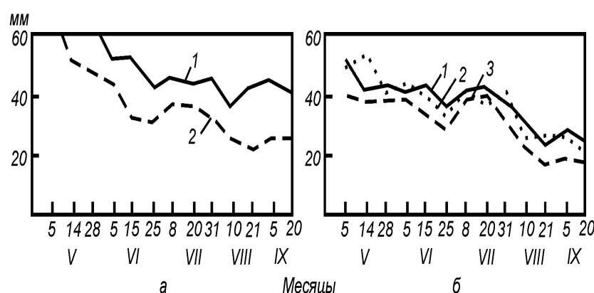
Рис. 16. Динамика запаса влаги, мм, в 50-сантиметровом слое почвы на вырубке и под пологом древостоя: а – северный склон; б – южный склон; 1 – вырубка; 2 – древостой; 3 – окно в древостое
