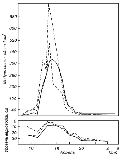
Рис. 11. Уровень верховодки и модуль весеннего стока в 1973 г. на Красноключевском стационаре (Башкирская АССР):
