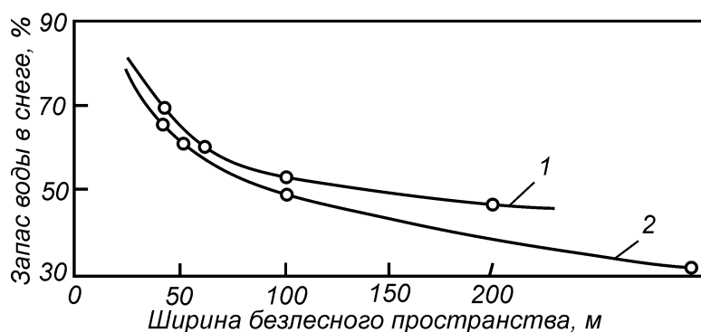
Рис. 8. Запас воды в снеге на безлесных площадях, % запаса на прогалинах, при ширине безлесного пространства: 1 – 500 м; 2 – 1000 м
