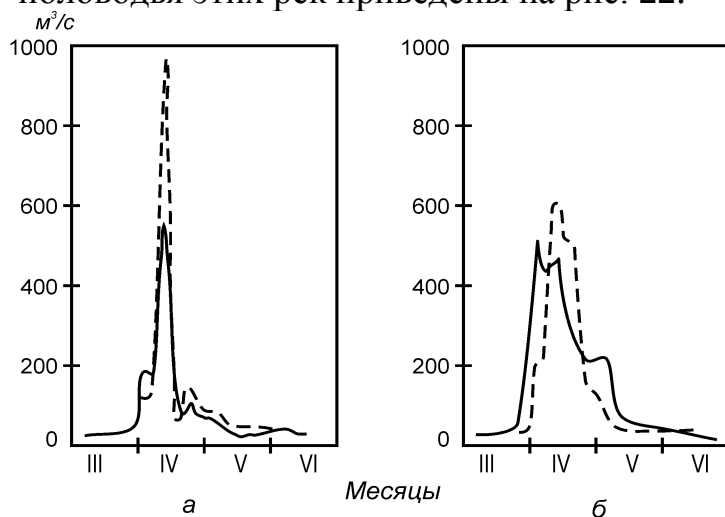
Рис. 22. Гидрографы половодий рек: а – Суры; б – Мокши; — 1938 г.; --- 1939 г.
