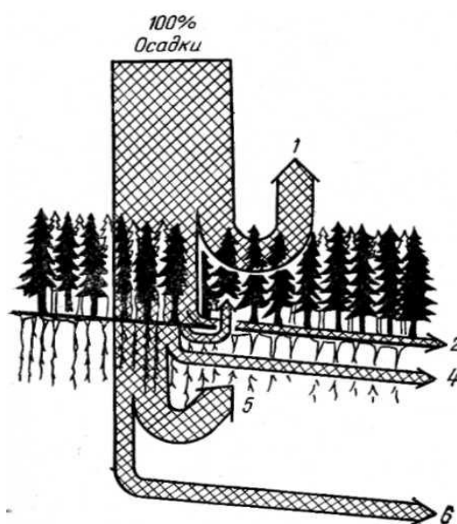
Рис. 9. Схема водного баланса почвы при водном режиме промывного типа (численные характеристики расходных статей баланса): 1 – задерживается кронами (30%); 2 – поверхностный сток (5%); 3 – физическое испарение и десукция напочвенным растительным покровом (10%); 4 – почвенный сток (10%); 5 – десукция древесным пологом (30%); 6 – грунтовой сток (15%)
