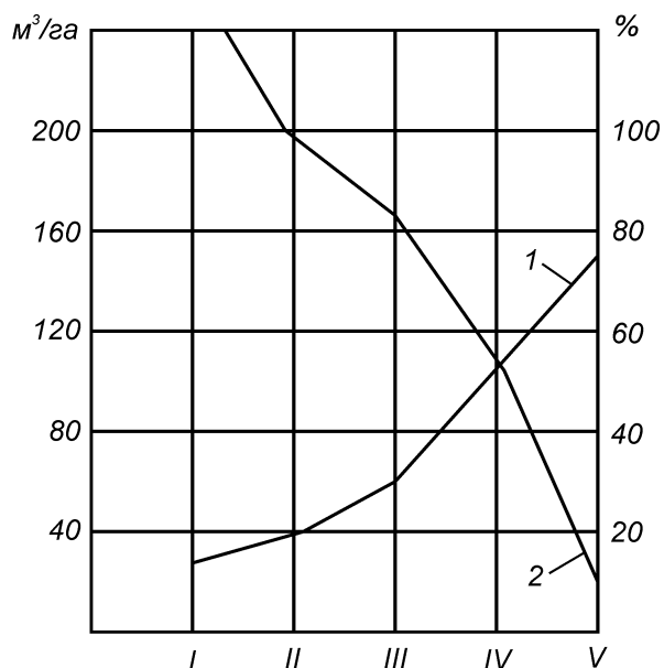
Рис. 19. Влияние на эрозию почвы способов трелевки в горных лесах Карпат (по Полякову, 1966) при спусках: I–V – соответственно наземном бессистемном, наземном лебедками, тракторном, гужевом бессистемном и подвесном; 1 – незеродированная часть поверхности почвы, %; 2 – вынос почвы, м 3 /га
