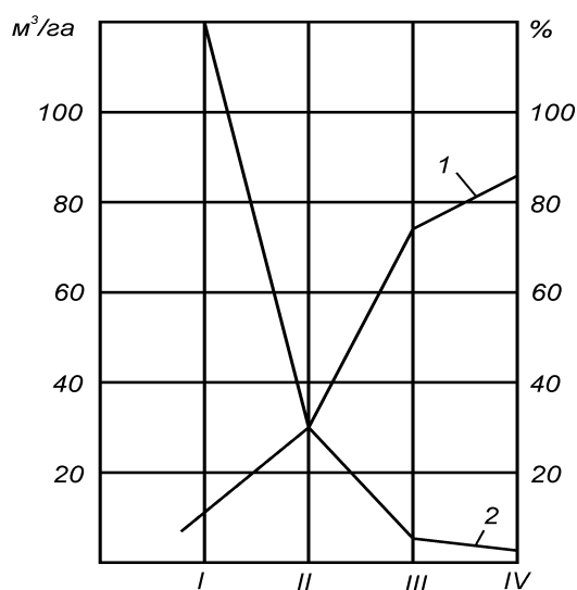
Рис. 18. Влияние на эрозию почвы рубок: I–IV – соответственно, сплошной, равномерно-постепенной, группово-постепенной и доброво-выборочной; 1 – неэродированная часть поверхности вырубки, %; 2 – вынос почвы, \text{м}^3/\text{га}
