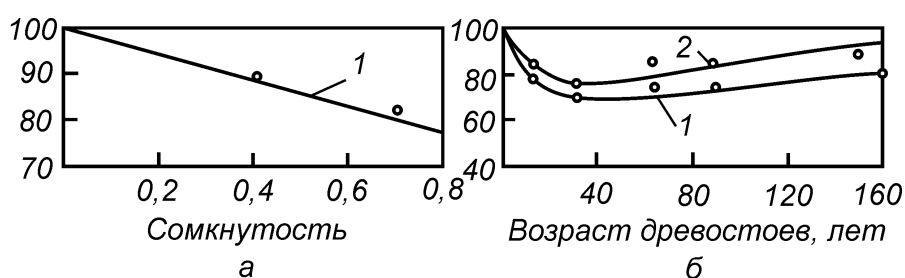
Рис. 6. Проникновение осадков под полог сосновых древостоев (по А. А. Молчанову, 1960) в зависимости: а – от сомкнутости; б – от возраста; 1 – дождь; 2 – снег
