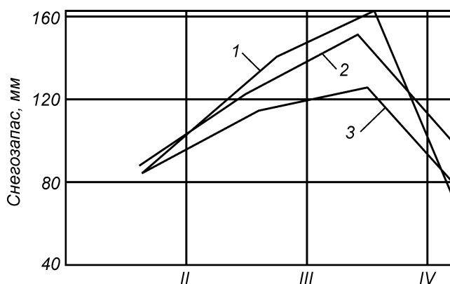
Рис. 20. Динамика снегозапасов в 1975 г.:
