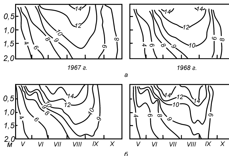
Рис. 4. Динамика температуры почвы (по А. Я. Орлову и др., 1974): а – в ельнике кислично-черничном; б – в сосняке мшисто-лишайниковом
