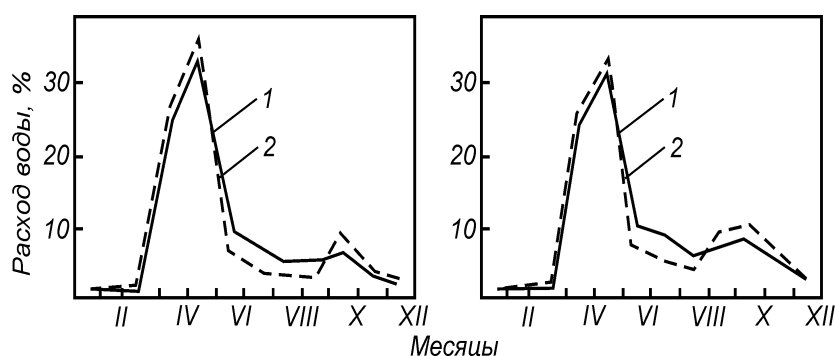
Рис. 21. Многолетний расход воды рек Большой Инзер (слева) и Малый Инзер: 1—1931–1947 гг.; 2—1918–1962 гг.
