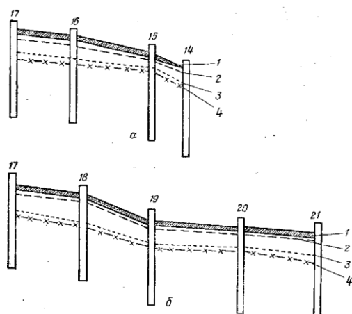
Рис. 10. Динамика верховодки на профилях Усьвинского стационара (Пермская обл.) при уровнях верховодки:
