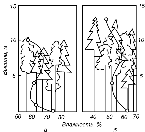
Рис. 2. Распределение относительной влажности воздуха в 13 ч (июль–август 1963г.) в молодняках при радиационном типе погоды (по В. В. Протопопову, 1975): а – елово-лиственных; б – кедрово-лиственных
