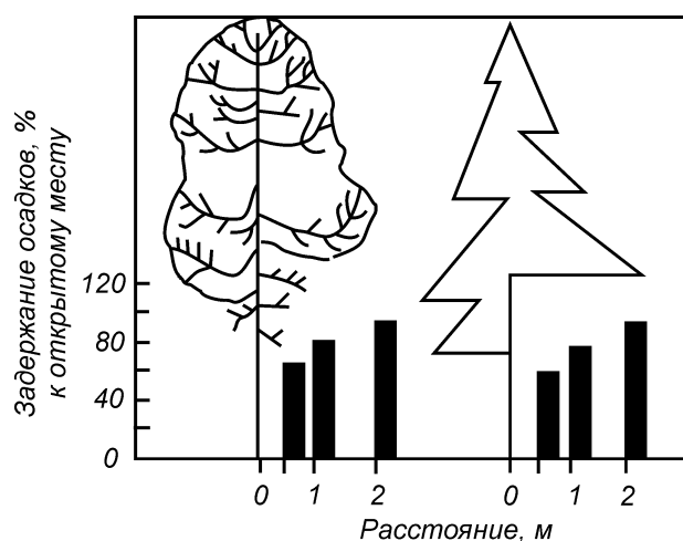
Рис. 7. Проникновение жидких осадков (средние величины за период с 1 июля по 31 августа 1961 г.) через кроны кедра (слева) и пихты на различных расстояниях от центра ствола (по В. В. Протопопову)
