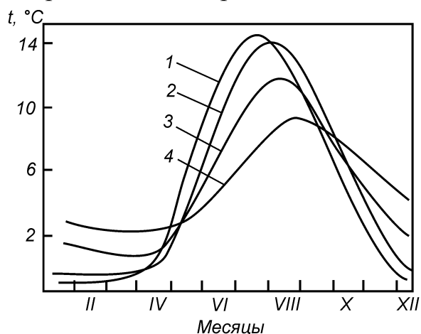
Рис. 3. Годовой ход температуры почвы в еловом лесу в 1967 г. (по А. Я. Орлову, 1974) на глубине:
