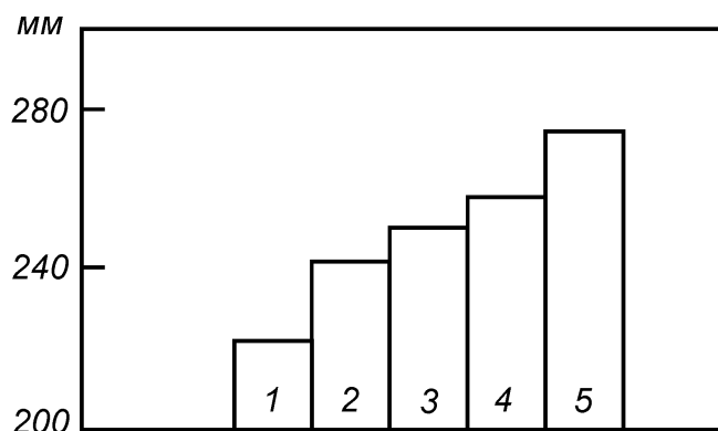
Рис. 17. Максимальные снегозапасы, мм: 1 – в лесу; 2–5 – соответственно, при выборочной, постепенной, сплошной концентрированной и узкополосной сплошной рубках
