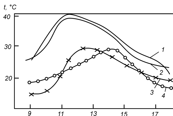
Рис. 5. Дневной ход температуры поверхности почвы (13 июля 1961 г.) в сосняке орляково-крупнотравном при различных способах ее подготовки: 1 – на пласту, 2 – при снятии дернины; 3 – на контроле; 4 – в борозде
