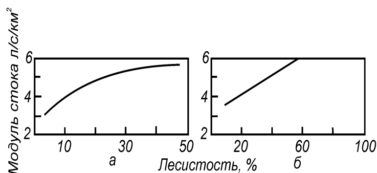
Рис. 13. График зависимости годового стока рек от лесистости бассейнов: а – верхнего Днепра и Оки (1936–1940 гг.); б – Вятки (1936–1939 гг.)
